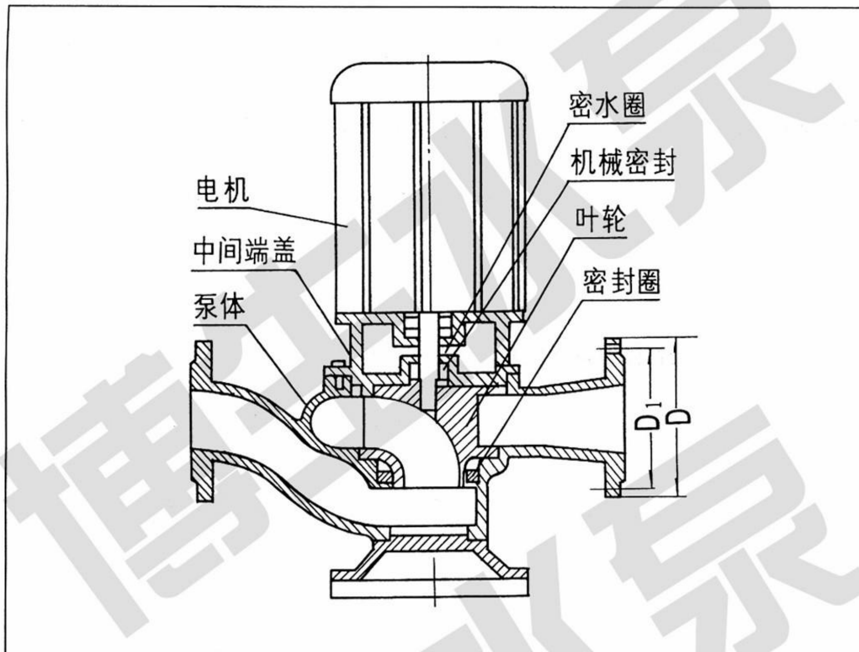
GW型管道排污泵结构图
